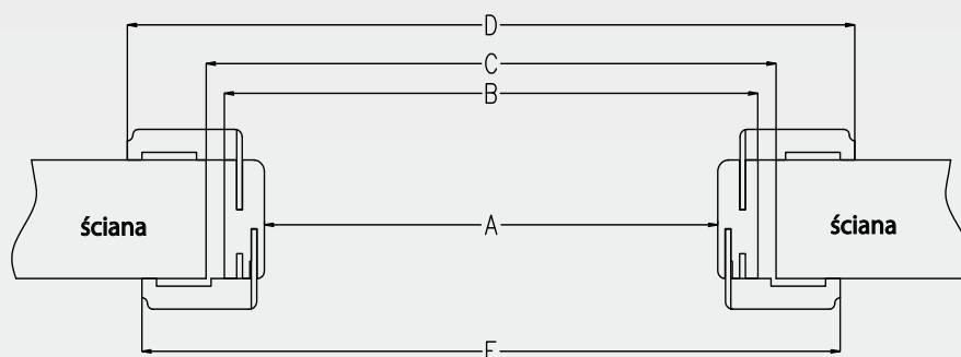
Tunel regulowany do drzwi pojedynczych
