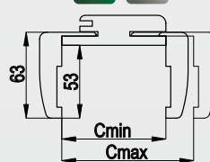
Przekrój ościeznicy regulowanej
