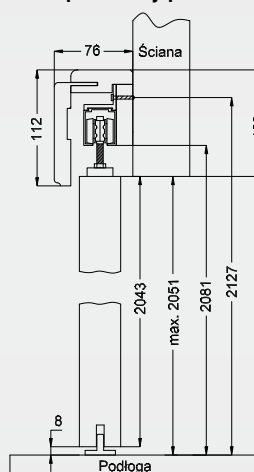
NS - przekrój pionowy
