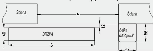
NS - przekrój poziomy
