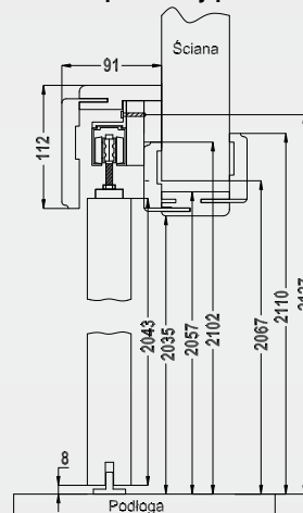
NT - przekrój pionowy
