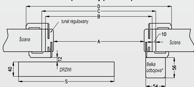
NT - przekrój poziomy
