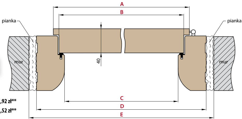
SCHEMAT OŚCIEŻNICY STAŁEJ
