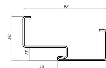
schemat ościeznicy
