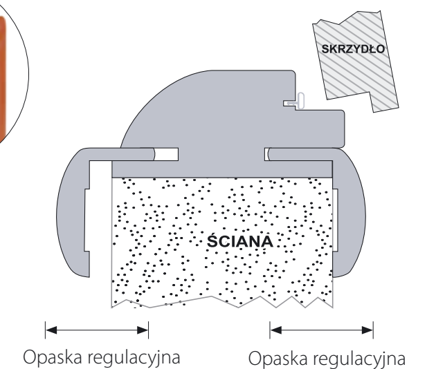
Schemat budowy ościeżnicy
