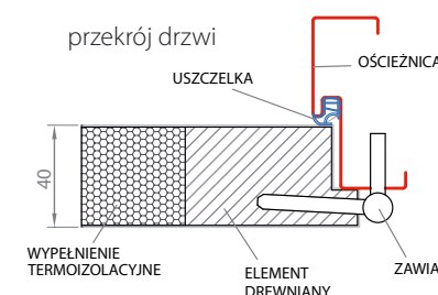
schemat ościeznicy
