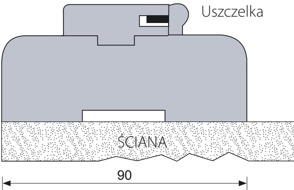
Schemat budowy ościeżnicy
