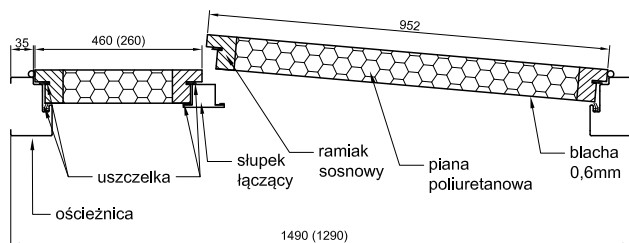
Przekrój poziomy przez drzwi dwuskrzydłowe
